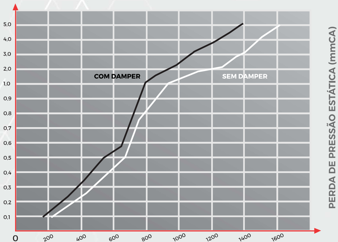
GRÁFICO DE VAZÃO DE AR (m³/h)
